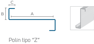
Polín tipo "Z"
