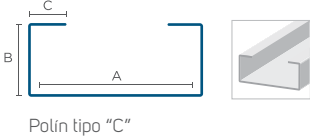
Polín tipo "C"
